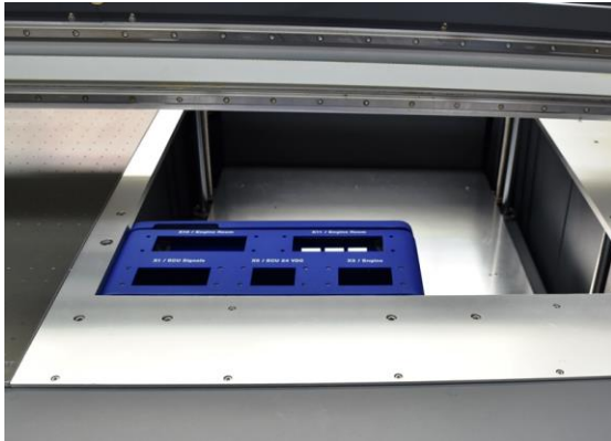
Höhenverstellbare Tischeinheit für die Bedruckung ganzer Gehäuse
