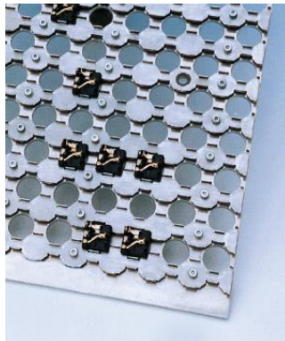
Werkstückträger Bereitstellung/Pufferung Relais
